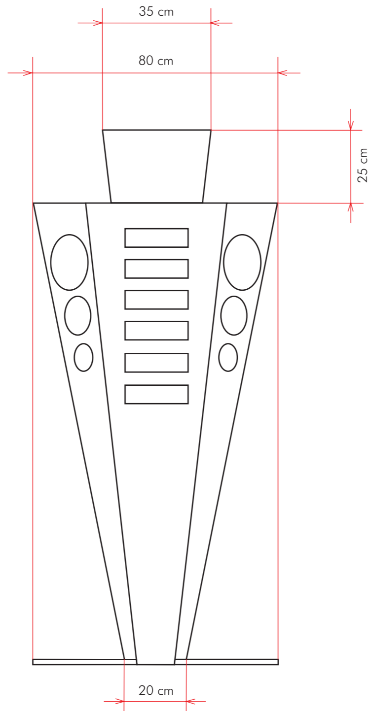
čelní pohled
