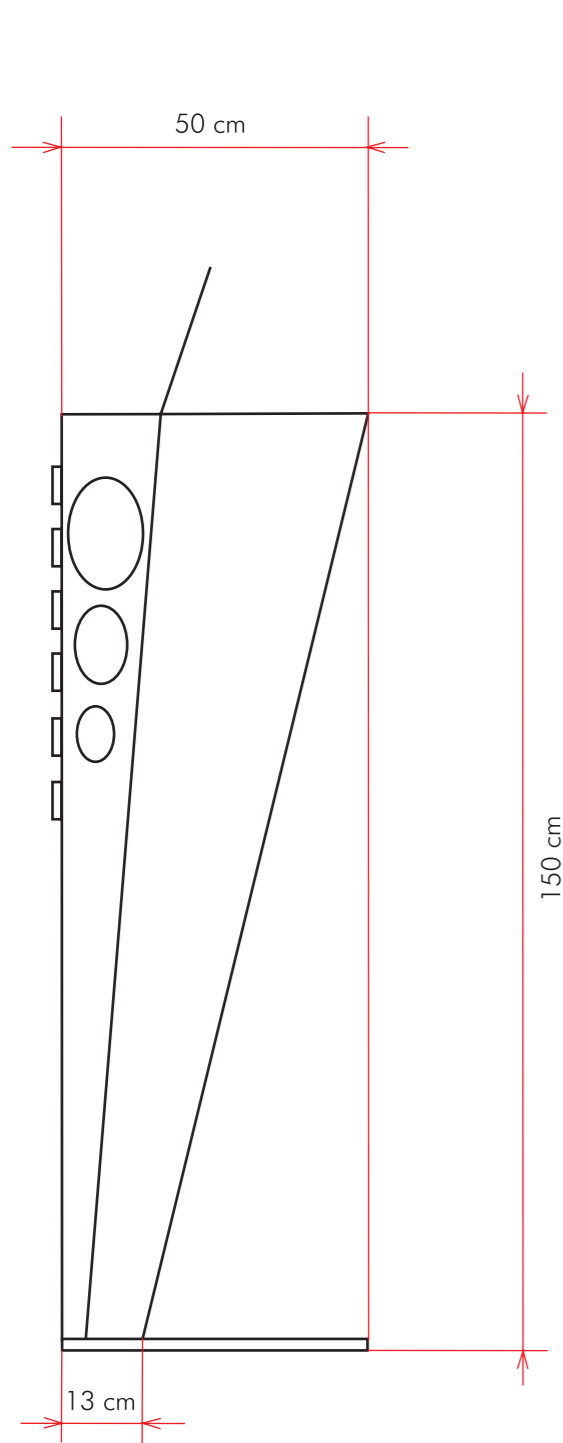
boční pohled
