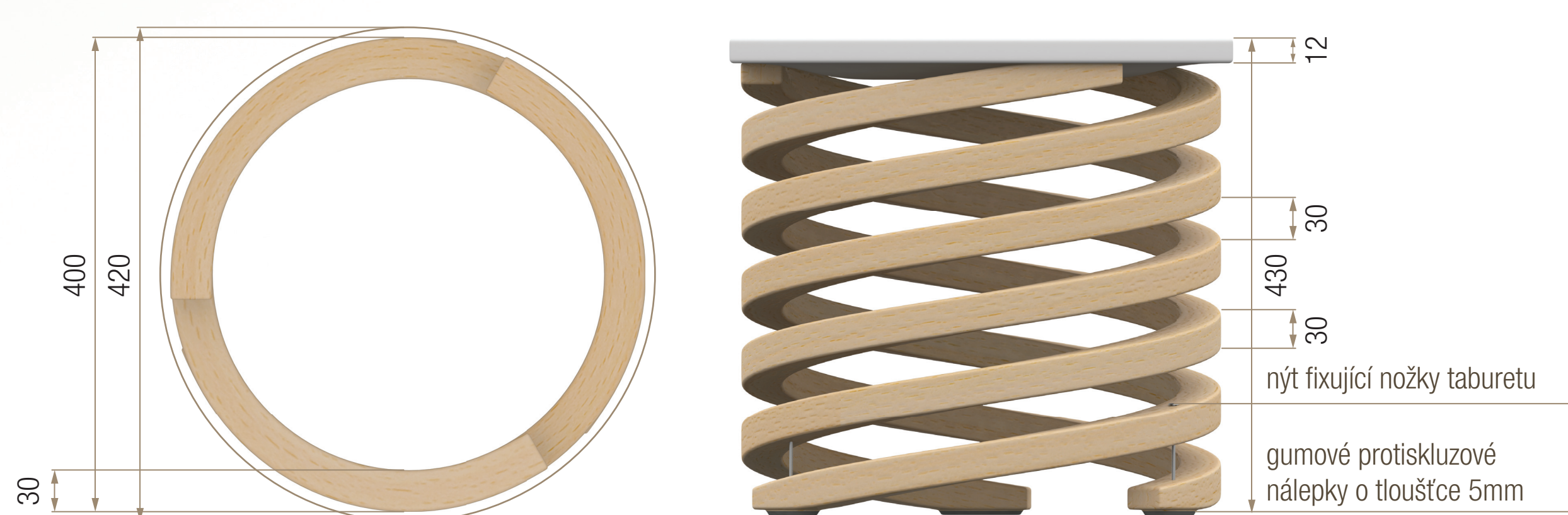
rozměry taburetu v mm
