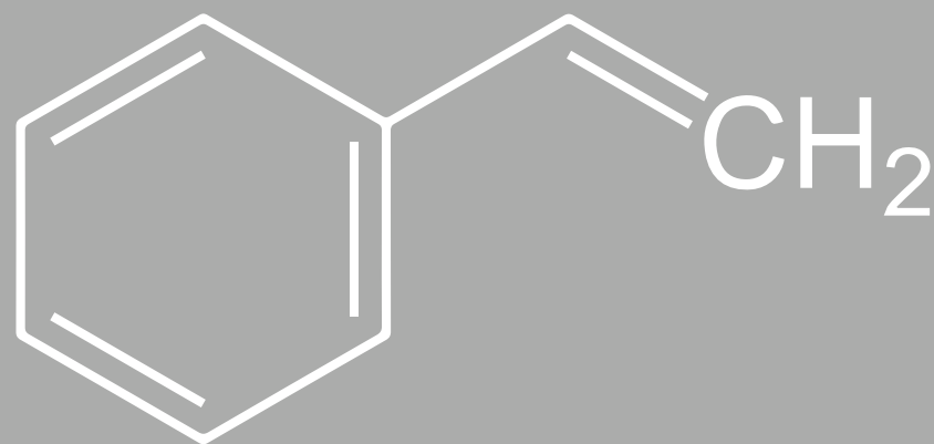
styrene
